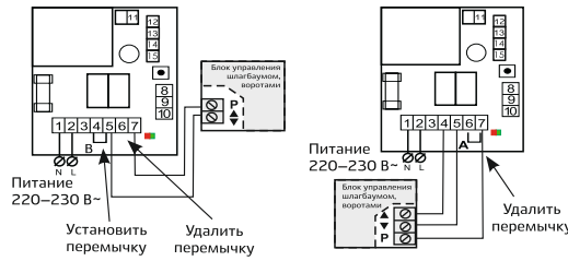
Рис. 2 — Подключение к пошаговому входу Рис. 3 — Подключение к раздельным входам «ОТКРЫТЬ» и «ЗАКРЫТЬ»
