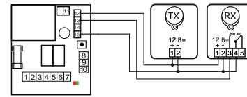
Рис. 6 — Подключение ИК-барьера
